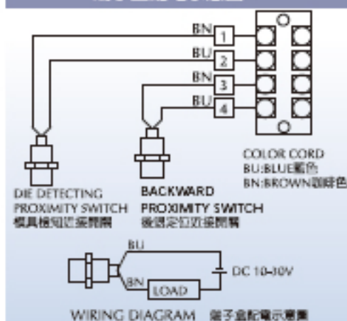
端子盒配電示意图
