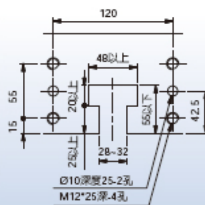
客戶台盤固定孔位及T槽尺寸範圍
